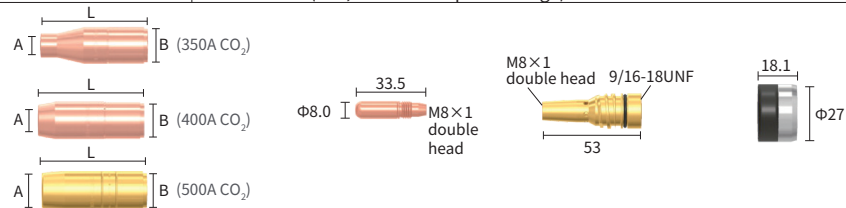
1-2-1.NOZZLE
